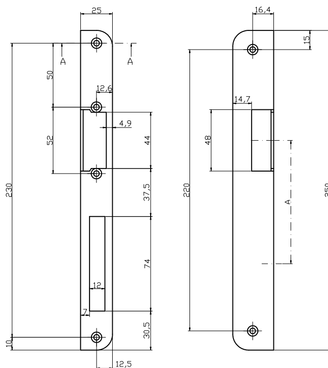
A=96,5 - wymiar między środkiem języka zamka a środkiem otworu podklamkowego
