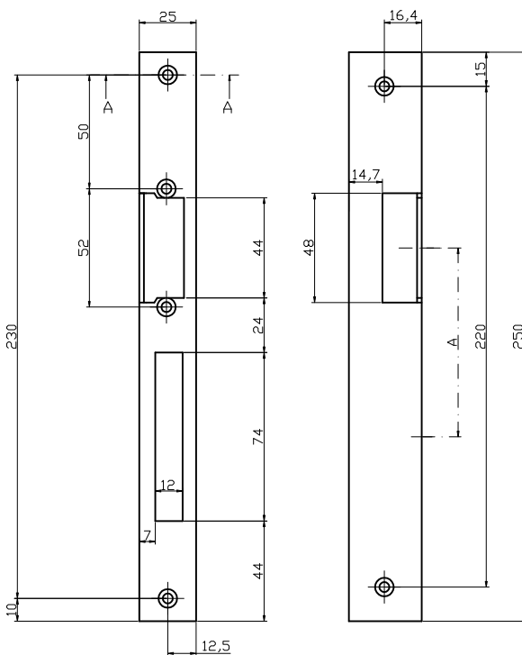
A=83 - wymiar między środkiem języka zamka a środkiem otworu podkławkowego
