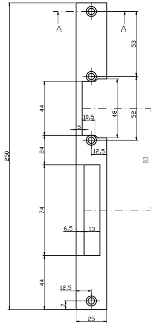
83 - wymiar między środkiem języka zamka a środkiem otworu podklamkowego
