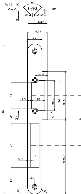
A=81,25 - wymiar między środkiem języka zamka a środkiem otworu podklamkowego
