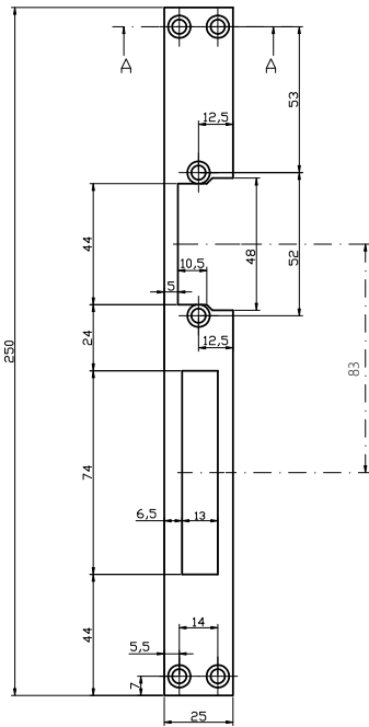
83 - wymiar między środkiem języka zamka a środkiem otworu podklamkowego
