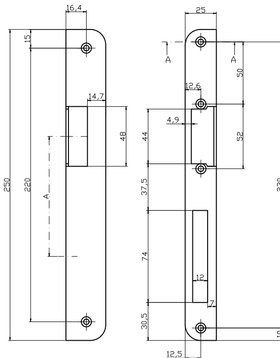
A=96,5 - wymiar między środkiem języka zamka a środkiem otworu podklamkowego
