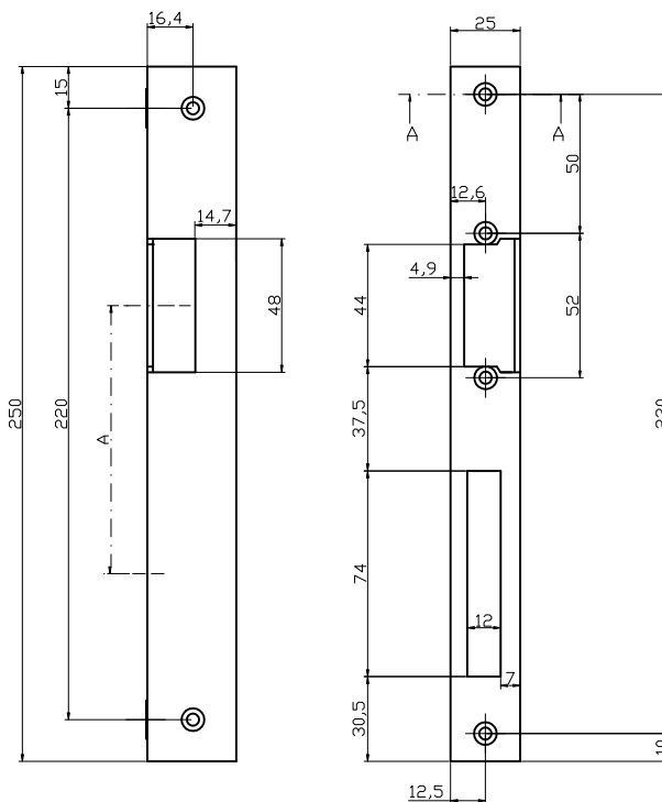
A=96,5 - wymiar między środkiem języka zamka a środkiem otworu podklamkowego
