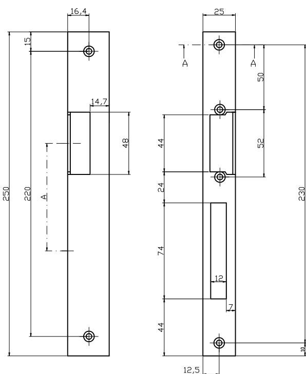
A=83 - wymiar między środkiem języka zamka a środkiem otworu podklamkowego
