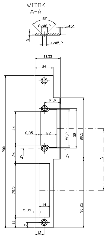
A=81,25 - wymiar między środkiem języka zamka a środkiem otworu podklamkowego
