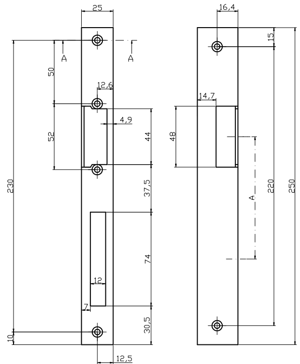
A=96,5 - wymiar między środkiem języka zamka a środkiem otworu podkławkowego
